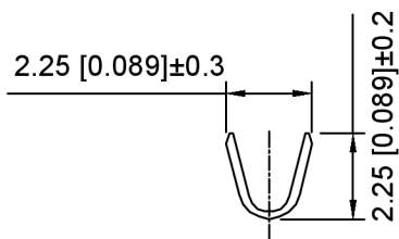
SEC:A-A
