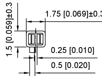
SEC:A-A
