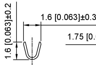
SEC:A-A
