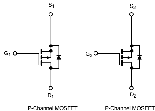
P-Channel MOSFET
