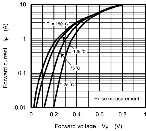
Fig. 10.1 I_F - V_F
