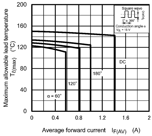
Fig. 10.4 T_{t(max)} - I_{F(AV)}
