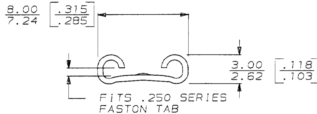
VIEW A-A
