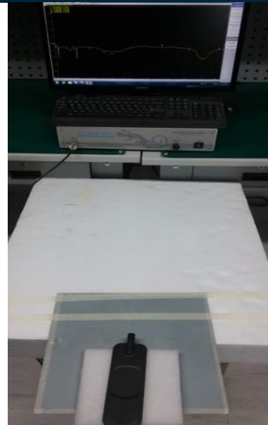
Antenna bent 90°
