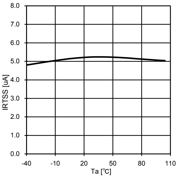
Fig.3 IRTSS-Ta (VRTSS=0V)
