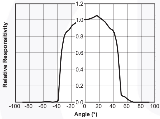
Fig. 3 Normalized Reception Pattern for the ALS Detector
