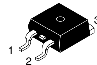
D 2 PAK-3 TO-263 CASE 418BK
