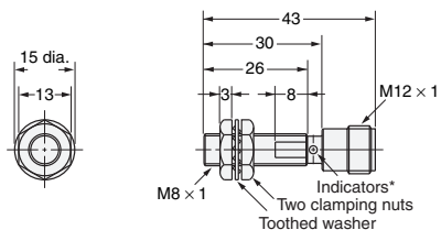
Diagram 18 E2E-X2D□-M1(G) E2E-X1R5E□-M1/E2E-X1R5F□-M1
