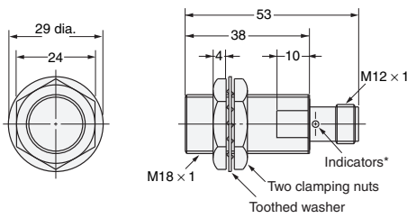
Diagram 24 E2E-X7D□-M1(G)/E2E-X5E□-M1/X5F□-M1 E2E-X5Y□-M1
