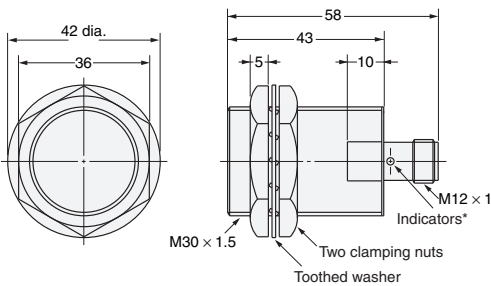
Diagram 26 E2E-X10D□-M1(G)/E2E-X10E□-M1/X10F□-M1 E2E-X10Y□-M1
