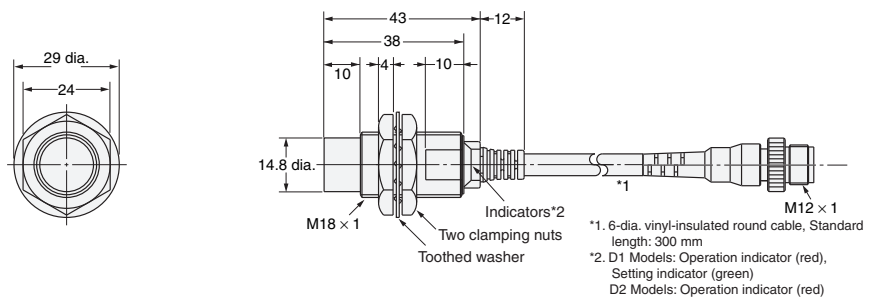
Diagram 34 E2E-X14MD□-M1GJ E2E-X14MD1-M1TGJ
