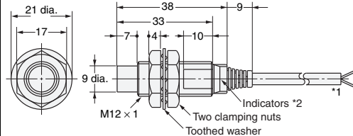
Diagram 10 E2E-X8MD□ E2E-X5ME□/F□
