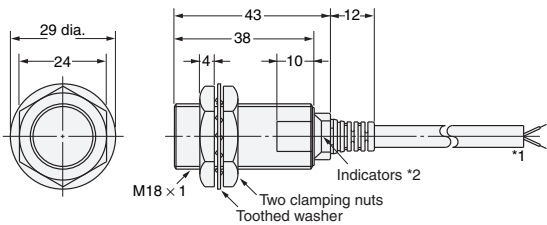
Diagram 14 E2E-X7D□/E2E-X5E□/F□ E2E-X5Y□/E2E-X7T1
