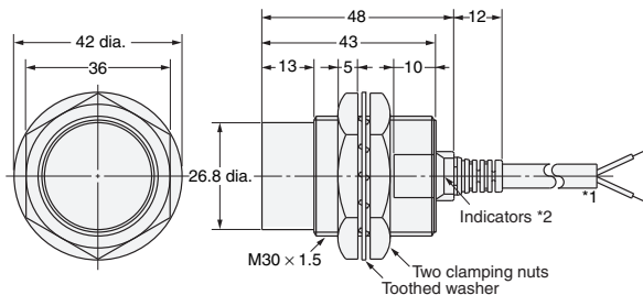
Diagram 17 E2E-X20MD□/E2E-X18ME□/F□ E2E-X18MY□
