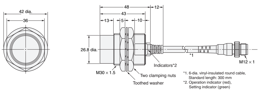
Diagram 36 E2E-X20MD1-M1GJ E2E-X20MD1-M1TGJ
