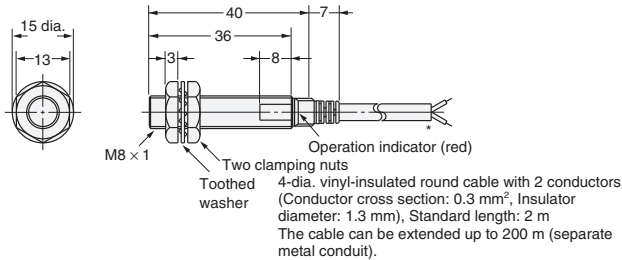
Diagram 9 E2E-X3D□ E2E-X2E□/F□
