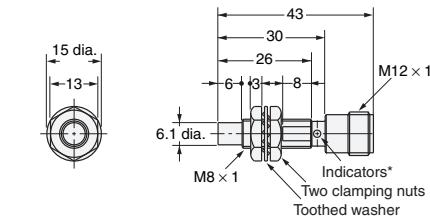
Diagram 19 E2E-X4MD□-M1(G) E2E-X2ME□-M1/E2E-X2MF□-M1
