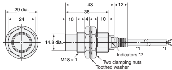
Diagram 15 E2E-X14MD□/E2E-X10ME□/F□ E2E-X10MY□
