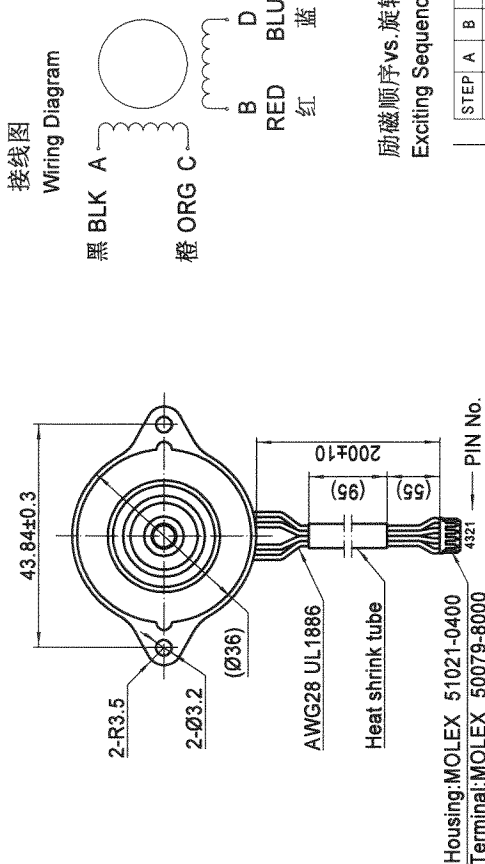
接线图 Wiring Diagram
