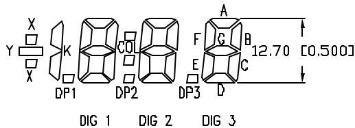
DIGIT DETAIL
