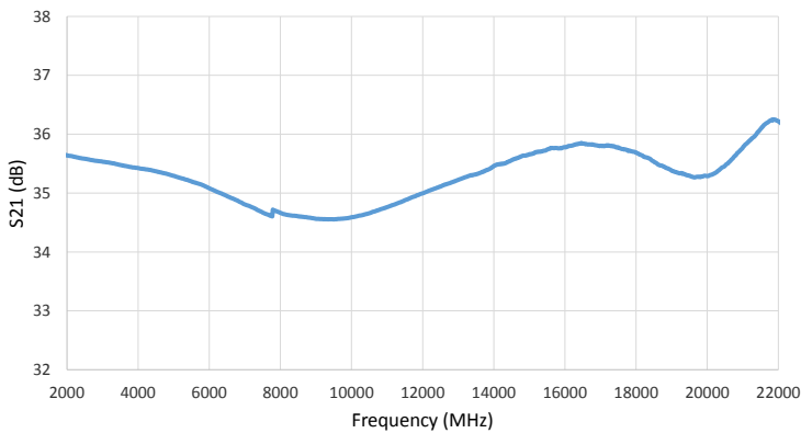
S21
