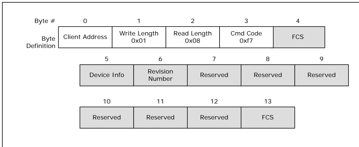
Figure 2-5. GetDIB()
