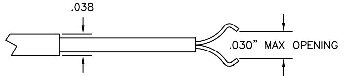
HOOK DETAIL 6X ACTUAL SIZE
