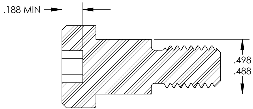
SECTION A-A
