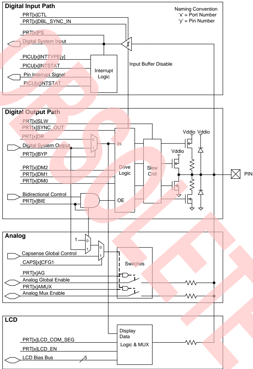
图 6-8. GPIO 框图
