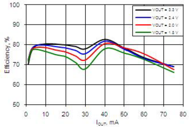
Figure 11-11. 效率与 I_{OUT} V_{BAT} 范围为 0.7\text{ V} 至 3.3\text{ V} , L_{BOOST} = 22\ \mu\text{H}
