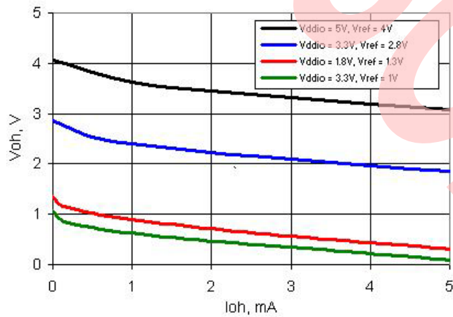
图 11-19. SIO 输出高电压和电流，稳压模式
