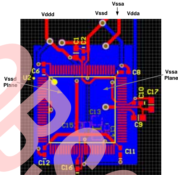
图 2-6. 100 引脚 TQFP 部件获得最佳模拟性能的 PCB 布局示例
