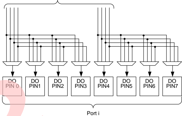
图 7-16. I/O 引脚输出连接
