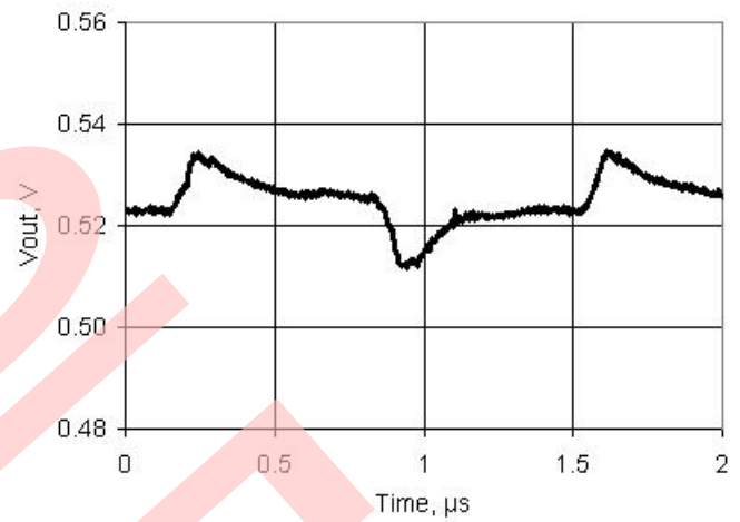
图 11-56. VDAC 脉冲响应，代码 0x7F - 0x80，1 V 模式，快速模式，V dda = 5 V
