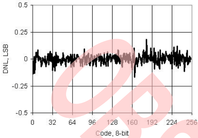
图 11-36. IDAC DNL 与输入代码, 范围 = 255 \mu A, 源电流模式
