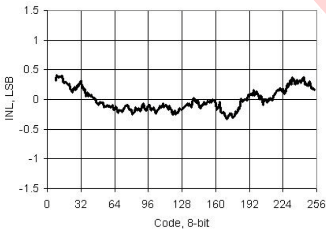
图 11-34. IDAC INL 与输入代码, 范围 = 255 \mu A, 源电流模式
