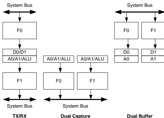
图 7-9. FIFO 配置示例
