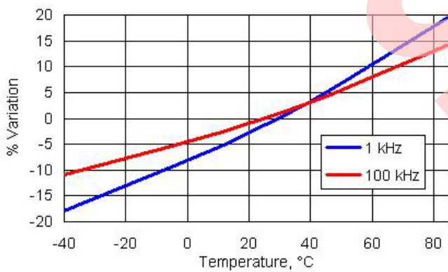
图 11-71. ILO 频率变化与温度
