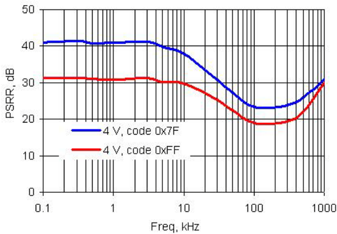
图 11-57. VDAC PSRR 与频率
