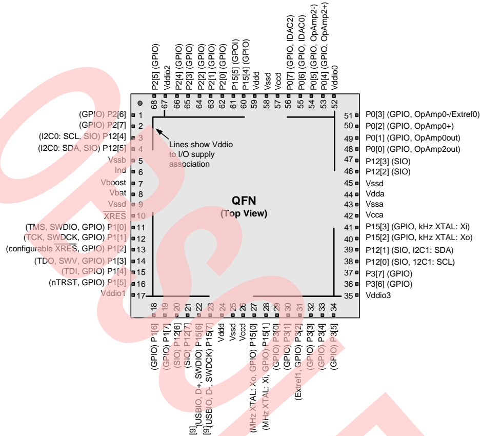
图 2-3. 68 引脚 QFN 部件的引脚分布图 [10]
