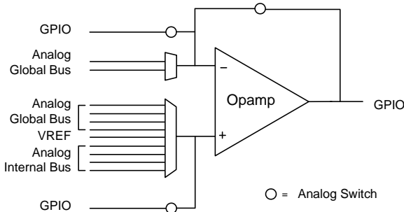
图 8-7. 运算放大器
