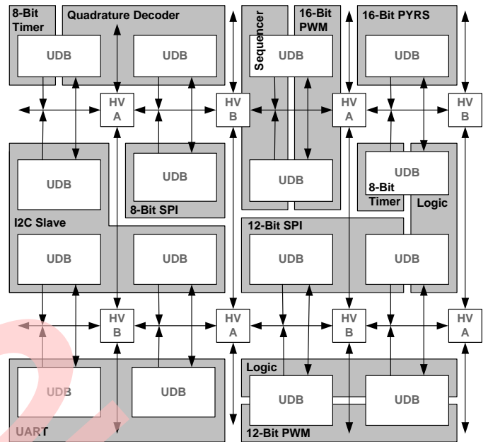
图 7-12. 一组 UDB 中的功能映射示例
