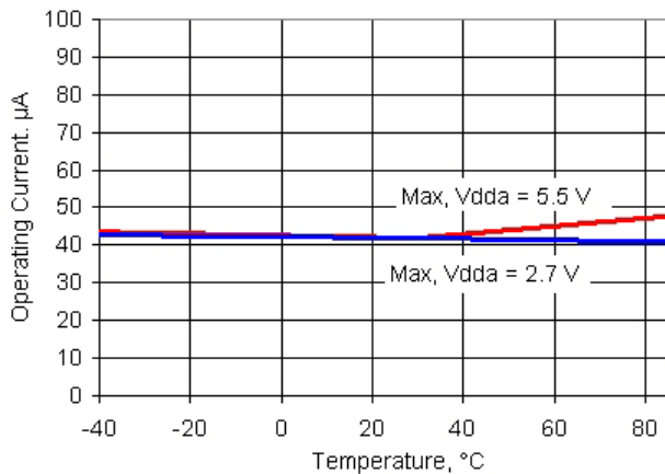
图 11-53. VDAC 工作电流与温度, 1V 模式, 慢速模式
