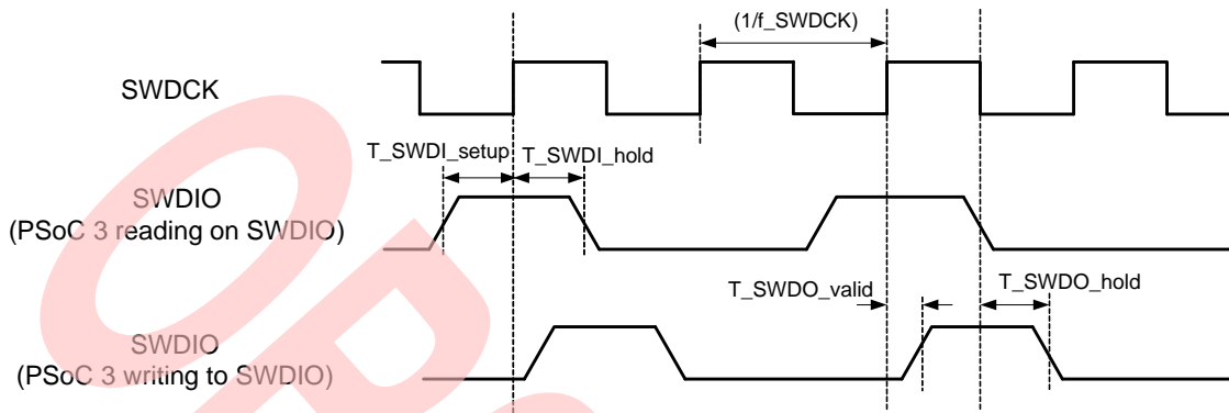
图 11-67. SWD 接口时序
