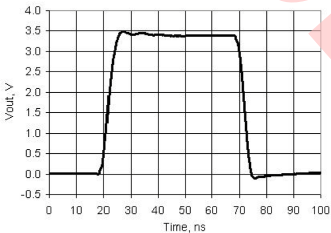
图 11-15. GPIO 输出上升和下降时间, 快速强 (Fast Strong) 驱动模式, V_{DDIO} = 3.3 V, 25 pF 负载
