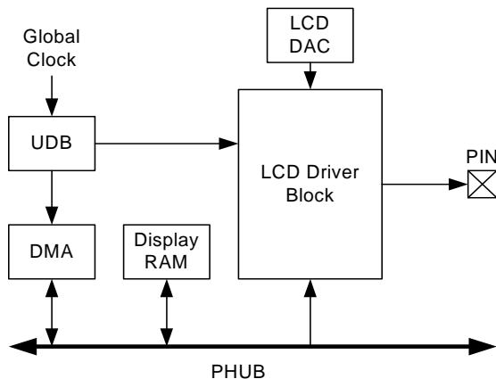
图 8-11. LCD 系统
