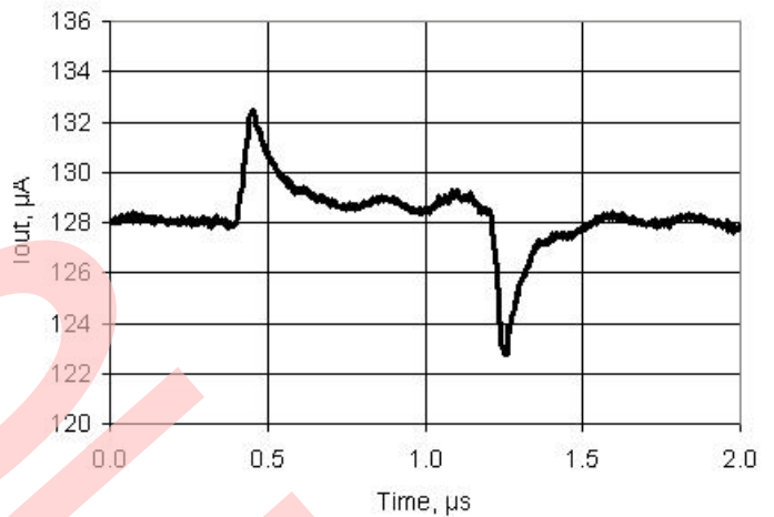
图 11-45. IDAC 脉冲响应, 代码 0x7F - 0x80, 255 \mu A 模式, 源电流模式, 快速模式, V_{DDA} = 5 V
