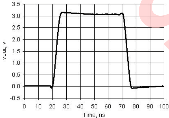
图 11-24. USBIO 输出上升和下降时间, GPIO 模式, V_{\text{DDD}} = 3.3\text{ V} , 25 pF 负载
