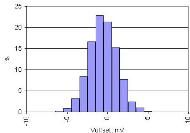
图 11-58. PGA 偏移柱状图，4096 采样 / 1024 部件
