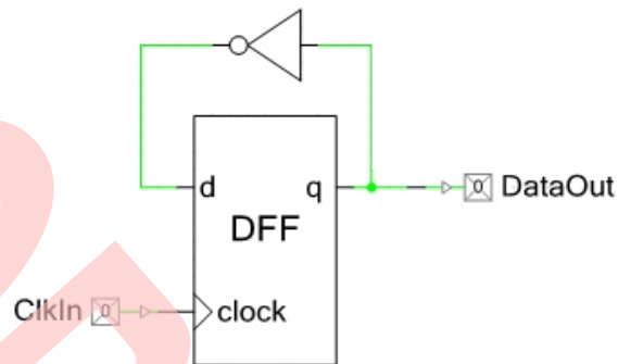
图 11-61. 时钟输入至数据输出方面的性能
