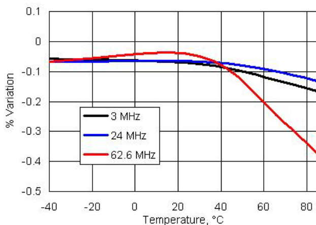
图 11-69. IMO 频率变化与温度
