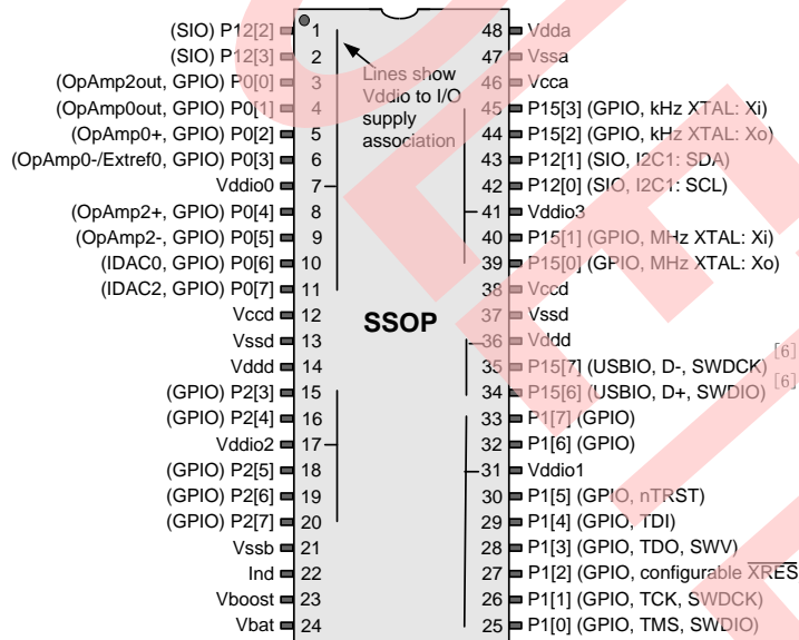
图 2-1. 48 引脚 SSOP 部件的引脚分布图
