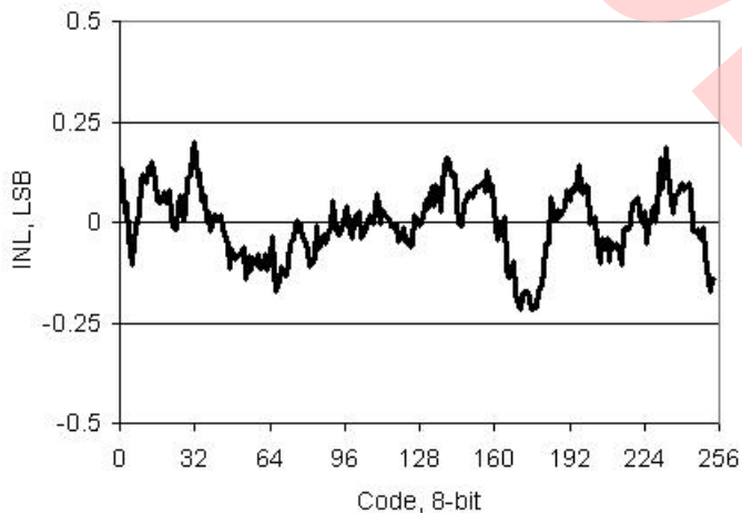
图 11-47. VDAC INL 与输出代码, 1V 模式
