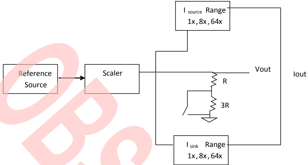
图 8-12. DAC 框图
