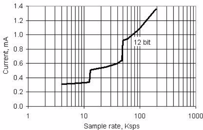
图 11-33. Delta-sigma ADC IDD 与 sps，范围 = ±1.024 V，连续采样模式，绕过输入缓冲区
