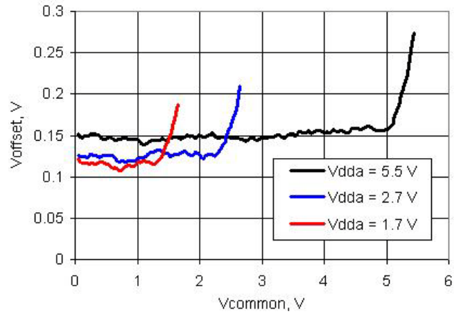
图 11-27. 运算放大器偏移与公用和 Vdda, 25 °C
