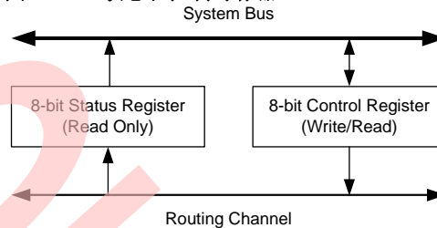
图 7-10. 状态和控制寄存器
