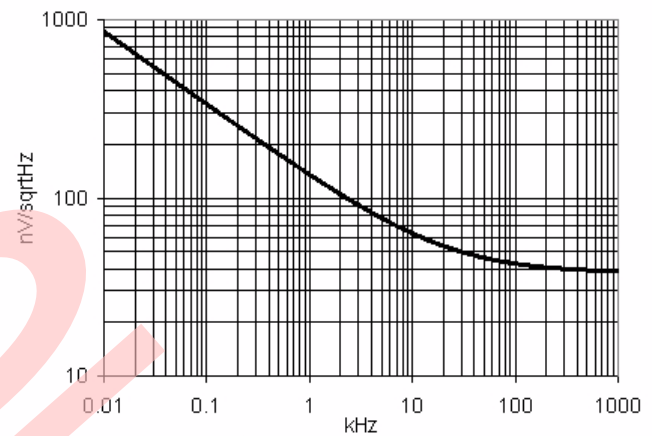
图 11-60. 噪声与频率, V_{DDA} = 5 V, 功耗模式 = 高
