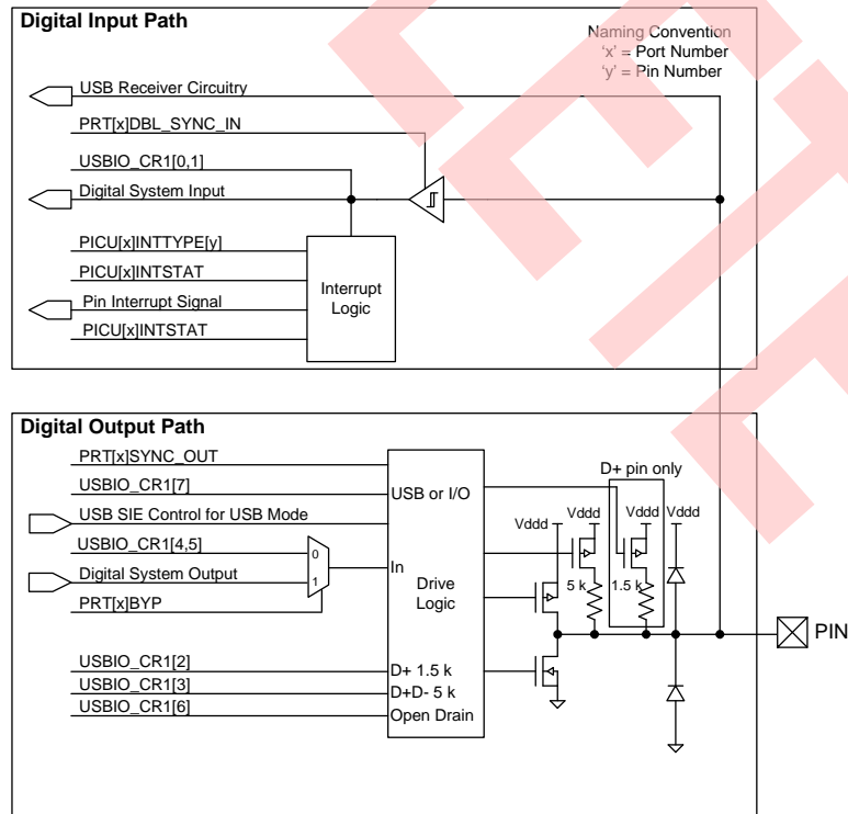
图 6-10. GPIO 框图
