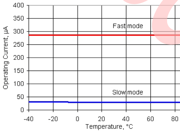
图 11-42. IDAC 工作电流与温度, 范围 = 255 \mu A, 代码 = 0, 源电流模式
