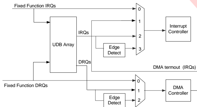
图 7-14. IDMUX 中的中断和 DMA 处理
