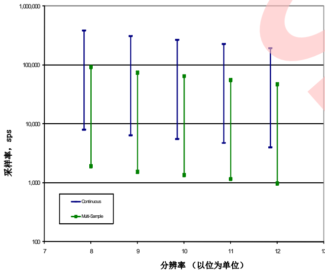
图 8-3. Delta-Sigma ADC 采样速率, 范围 = ±1.024 V
