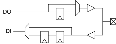
图 7-15. I/O 引脚同步路由
