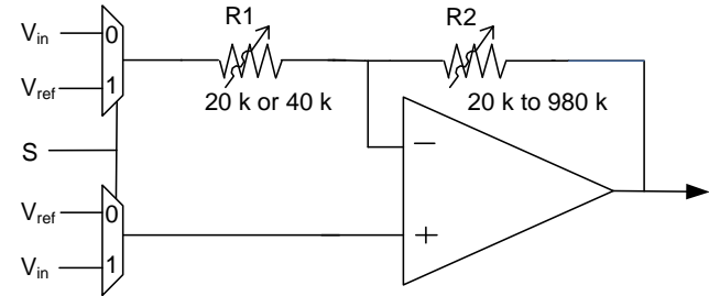
图 8-9. PGA 电阻设置
