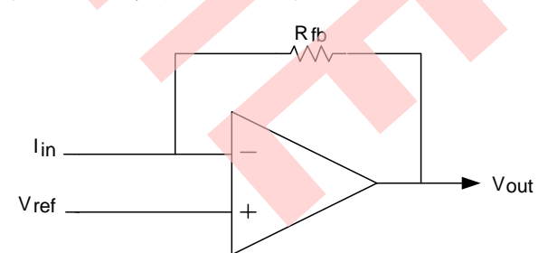
图 8-10. 连续时间 TIA 原理图
