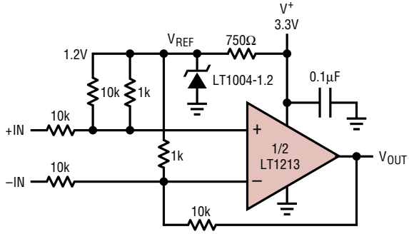
1213/14 TA05
